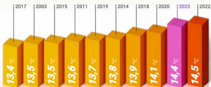
LES 10 ANNÉES LES PLUS CHAUDES EN FRANCE DEPUIS 1900
