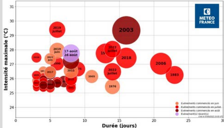
Vagues de chaleur observées
